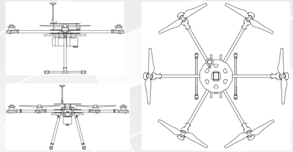
HEXACÓPTERO PROFESIONAL ÁGUILA-6
